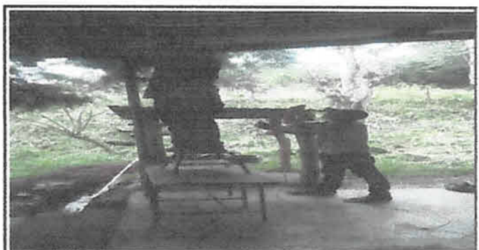
Foto 6: Reparación del sistema eléctrico para el modulo 3 del salón I con puesta de 1 plafonera, 2 tomacorrientes y 1 apagador.
